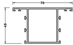
TB-2252 (1,062 kg/mt) GENİŞ ORTA KAYIT PROFİLİ
