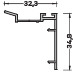
TB-3023 (0,267 kg/mt) DAR KENET PROFİLİ
