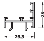
TB-3022 (0,333 kg/mt) DAR ADAPTÖR PROFİLİ
