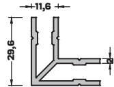
TB-3034 (0,238 kg/mt) GENİŞ ALT RAY PROFİLİ
