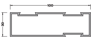
TB-3711 (0,711 kg/mt) SİNEKLİK KANAT PROFİLİ
