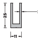
TB-141 (0,346 kg/mt) DAR 'U' BAĞLANTI PROFİLİ
