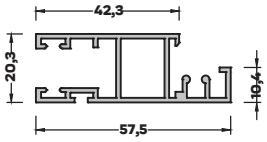
TB-3711 (0,711 kg/mt) SİNEKLİK KANAT PROFİLİ
