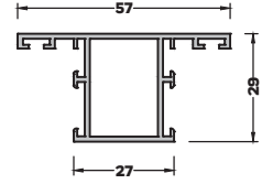
TB-3028 (0,631 kg/mt) DAR ORTA PROFİLİ
