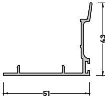
TB-3033 (0,444 kg/mt) GENİŞ KENET PROFİLİ
