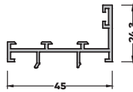
TB-3032 (0,413 kg/mt) GENİŞ ADAPTÖR PROFİLİ
