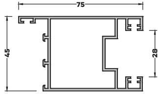
TB-3031 (1,161 kg/mt) GENİŞ KANAT PROFİLİ
