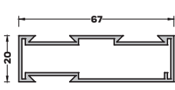
TB-3020 (0,715 kg/mt) DAR KASA PROFİLİ
