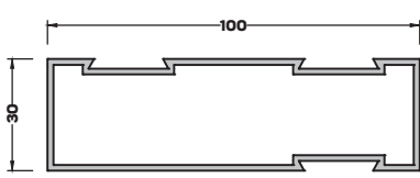
TB-3711 (0,711 kg/mt) SİNEKLİK KANAT PROFİLİ
