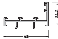
TB-3032 (0,413 kg/mt) GENİŞ ADAPTÖR PROFİLİ
