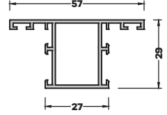
TB-3028 (0,631 kg/mt) DAR ORTA PROFİLİ
