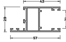
TB-3021 (0,680 kg/mt) DAR KANAT PROFİLİ
