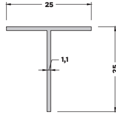
T-156 (0,146 kg/mt) T BİNİ PROFİLİ
