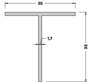
T-4233(0,314 kg/mt) T BİNİ PROFİLİ
