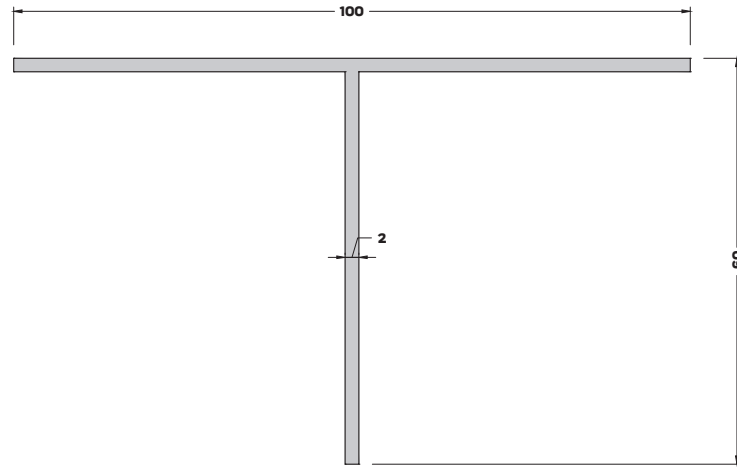
T-7206 (0,853 kg/mt) T BİNİ PROFİLİ
