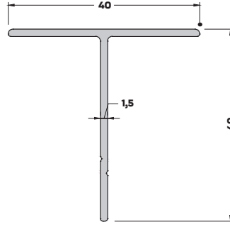
T-4690 (0,320 kg/mt) T BİNİ PROFİLİ
