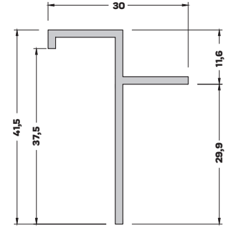
T-11484 (0,320 kg/mt) ASİMETRİK T BİNİ PROFİLİ
