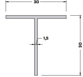
T-1183 (0,273 kg/mt) T BİNİ PROFİLİ
