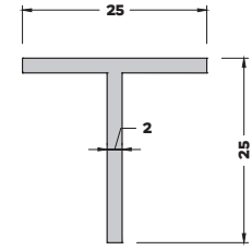
T-1183 (0,273 kg/mt) T BİNİ PROFİLİ
