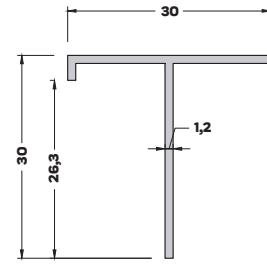
T-5575 (0,205 kg/mt) T BİNİ PROFİLİ
