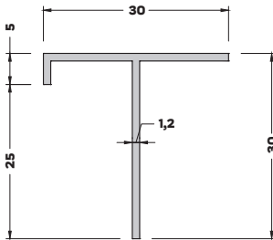
T-6341 (0,176 kg/mt) T BİNİ PROFİLİ
