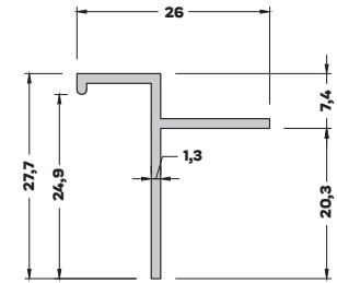
T-1512 (0,180 kg/mt) ASİMETRİK T BİNİ PROFİLİ
