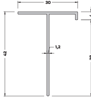
T-1035 (0,239 kg/mt) T BİNİ PROFİLİ
