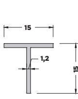
T-4681 (0,093 kg/mt) T BİNİ PROFİLİ
