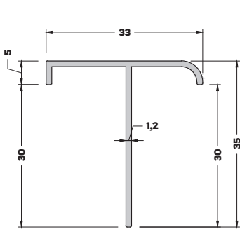
T-1139 (0,239 kg/mt) T BİNİ PROFİLİ
