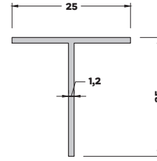
T-3062(0,158 kg/mt) T BİNİ PROFİLİ
