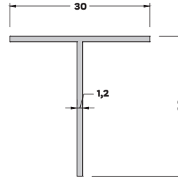
T-3062(0,158 kg/mt) T BİNİ PROFİLİ
