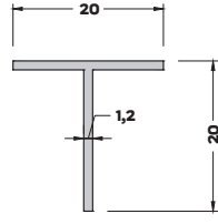
T-4680(0,126 kg/mt) T BİNİ PROFİLİ
