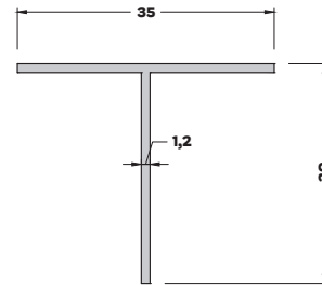
T-3063(0,176 kg/mt) T BİNİ PROFİLİ
