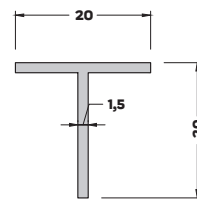
T-706(0,160 kg/mt) T BİNİ PROFİLİ
