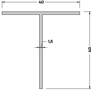
T-2969 (0,324 kg/mt) T BİNİ PROFİLİ
