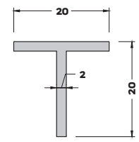
T-3265 (0,463 kg/mt) T BİNİ PROFİLİ
