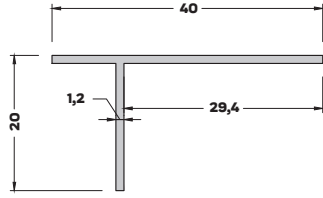
T-2969 (0,324 kg/mt) T BİNİ PROFİLİ
