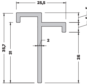
T-1123 (0,355 kg/mt) ASİMETRİK T BİNİ PROFİLİ
