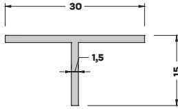
T-6341 (0,176 kg/mt) T BİNİ PROFİLİ
