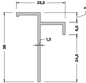
T-1121 (0,232 kg/mt) ASİMETRİK T BİNİ PROFİLİ
