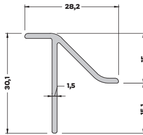
T-266 (0,250 kg/mt) ASİMETRİK T BİNİ PROFİLİ
