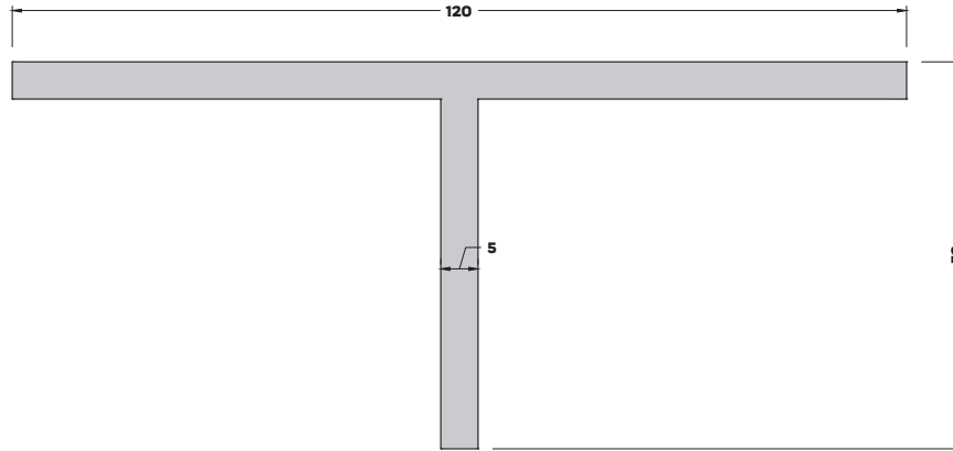
T-7206 (0,853 kg/mt) T BİNİ PROFİLİ
