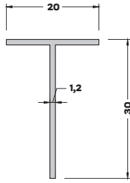
T-704 (0,160 kg/mt) T BİNİ PROFİLİ
