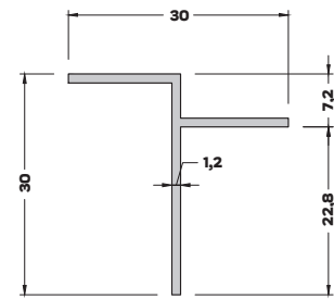
T-5527 (0,200 kg/mt) ASİMETRİK T BİNİ PROFİLİ
