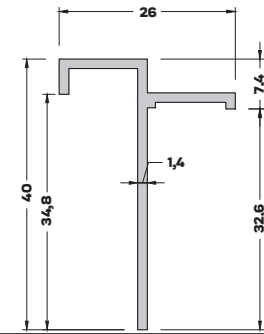
T-1555 (0,270 kg/mt) ASİMETRİK T BİNİ PROFİLİ
