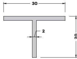
T-1756 (0,273 kg/mt) T BİNİ PROFİLİ
