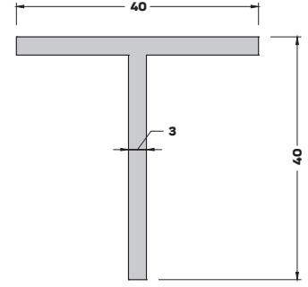
T-8276 (0,626 kg/mt) T BİNİ PROFİLİ
