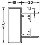
SN-4330 (0,528 kg/mt) SİNEKLİK DİKME PROFİLİ
