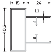
SN-4331 (0,520 kg/mt) SİNEKLİK DİKME PROFİLİ
