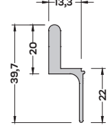
SN-4108 (0,442 kg/mt) SİNEKLİK PROFİLİ
