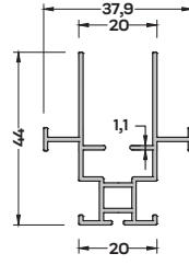
SN-4332 (0,516 kg/mt) SİNEKLİK KANAT PROFİLİ
