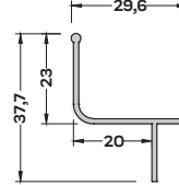
SN-1490 (0,227 kg/mt) SİNEKLİK PROFİLİ
