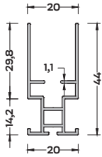
SN-4822 (0,421 kg/mt) SİNEKLİK KANAT PROFİLİ
