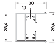
SN-4332 (0,427 kg/mt) SİNEKLİK RAY PROFİLİ
