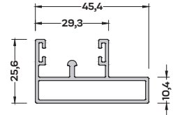
SN-1462 (0,391 kg/mt) SİNEKLİK RAY PROFİLİ
