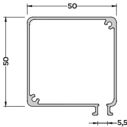
SN-3926 (0,804 kg/mt) SİNEKLİK PROFİLİ
