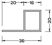
SN-3277 (0,309 kg/mt) SİNEKLİK KASA PROFİLİ
