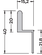
SN-5967 (0,222 kg/mt) SİNEKLİK PROFİLİ
