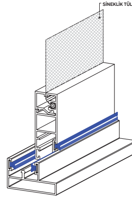
SN-6232 (0,499 kg/mt) SİNEKLİK KANAT PROFİLİ
