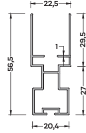
SN-6232 (0,499 kg/mt) SİNEKLİK KANAT PROFİLİ
