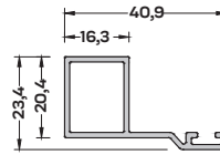
SN-2285 (0,370 kg/mt) SİNEKLİK RAY PROFİLİ
