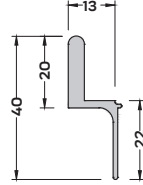
SN-4107 (0,282 kg/mt) SİNEKLİK PROFİLİ
