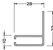
SN-1437 (0,316 kg/mt) SİNEKLİK F PROFİLİ
