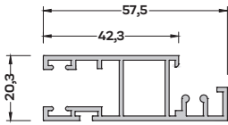
SN-2780 (0,400 kg/mt) SİNEKLİK PROFİLİ
