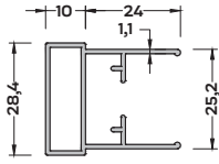
SN-4330 (0,528 kg/mt) SİNEKLİK DİKME PROFİLİ
