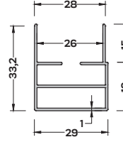
SN-6231 (0,383 kg/mt) SİNEKLİK RAY PROFİLİ
