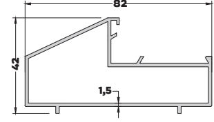
AB-4476 (0,965 kg/mt) KAPI KASA PROFİLİ
