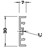
AB-6635 (0,203 kg/mt) KAPAK PROFİLİ
