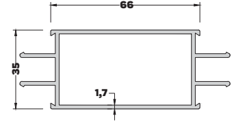
AB-4476 (0,965 kg/mt) KAPI KASA PROFİLİ
