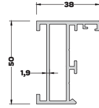
AB-6543 (0,944 kg/mt) PST SİSTEM KASA PROFİLİ
