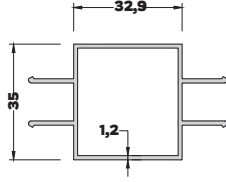
AB-1843 (0,756 kg/mt) TAŞIYICI GÖVDE PROFİLİ
