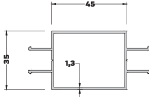
AB-2702 (0,740 kg/mt) TAŞIYICI GÖVDE PROFİLİ
