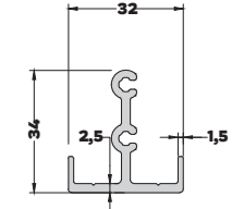
AB-11272 (0,560 kg/mt) ARA BÖLME BAĞLANTI PROFİLİ
