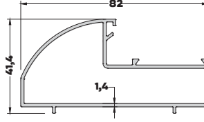
AB-6545 (0,912 kg/mt) KAPI KASA PROFİLİ
