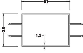
AB-1843 (0,756 kg/mt) TAŞIYICI GÖVDE PROFİLİ
