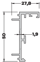
AB-6541 (0,556 kg/mt) ADAPTÖR PROFİLİ
