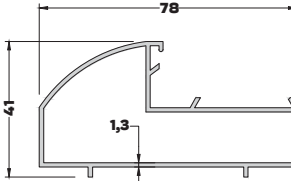
AB-6635 (0,203 kg/mt) KAPAK PROFİLİ
