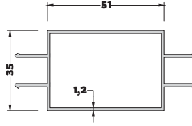
AB-6545 (0,912 kg/mt) KAPI KASA PROFİLİ
