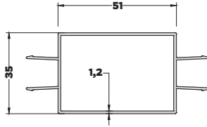
AB-6637 (0,692 kg/mt) TAŞIYICI GÖVDE PROFİLİ
