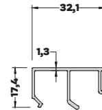
AB-11272 (0,560 kg/mt) ARA BÖLME BAĞLANTI PROFİLİ
