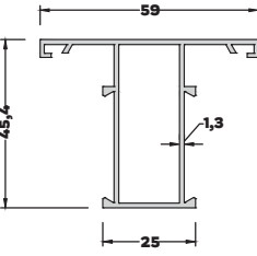
AL-220 (0,711 kg/mt) GENİŞ KASA PROFİLİ
