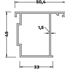
AL-3039 (0,744 kg/mt) PİVOT ADAPTÖR PROFİLİ
