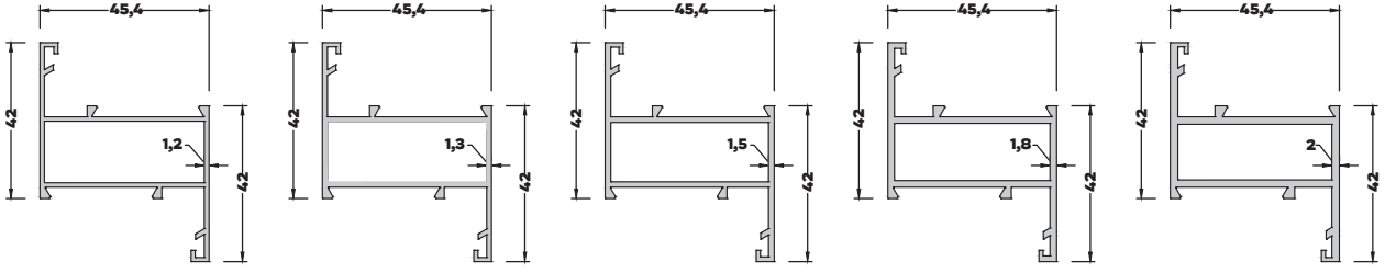
AL-3079 (0,653 kg/mt) DAR KANAT PROFİLİ
