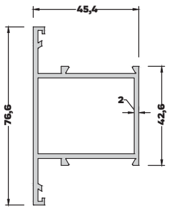
AL-209 (0,997 kg/mt) DAR ORTA KAYIT PROFİLİ
