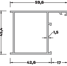
AL-244 (0,809 kg/mt) GENİŞ KASA PROFİLİ
