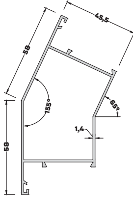
AL-2636 (1,083 kg/mt) 155° KÖŞE DÖNÜŞ PROFİLİ
