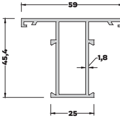
AL-280 (0,959 kg/mt) GENİŞ KASA PROFİLİ
