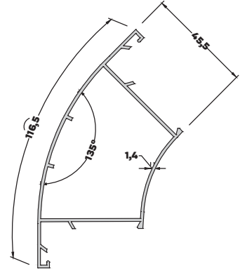
AL-3645 (0,985 kg/mt) 45° DÖNÜŞ PROFİLİ
