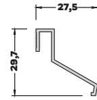
AL-3047 (0,246 kg/mt) DAMLALIK PROFİLİ
