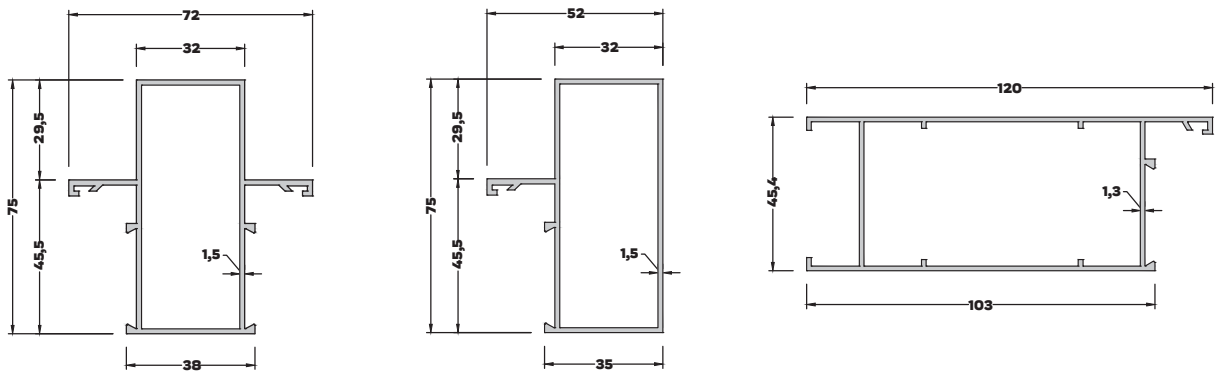
AL-3087 (1,144 kg/mt) TEKVİYELİ ORTA KAYIT PR.
