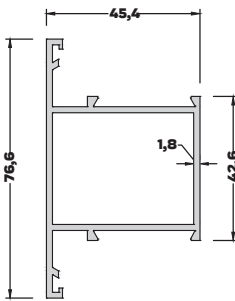
AL-281 (0,916 kg/mt) DAR ORTA KAYIT PROFİLİ
