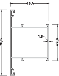
AL-221 (0,693 kg/mt) DAR ORTA KAYIT PROFİLİ
