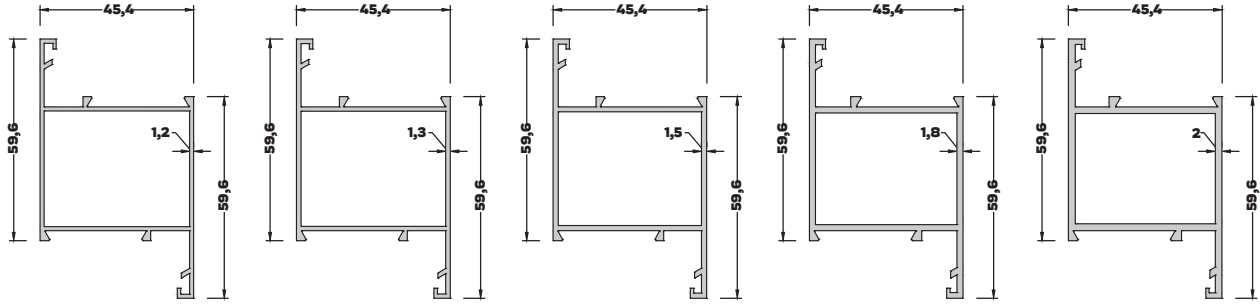
AL-3075 (0,767 kg/mt) GENİŞ KANAT PROFİLİ
