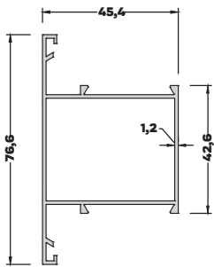
AL-3078 (0,658 kg/mt) DAR ORTA KAYIT PROFİLİ
