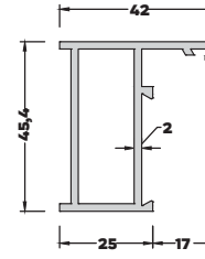
AL-211 (0,858kg/mt) DAR KASA PROFİLİ
