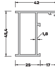
AL-283 (0,783 kg/mt) DAR KASA PROFİLİ
