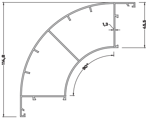
AL-3908 (1,582 kg/mt) 90° KÖŞE DÖNÜŞ PROFİLİ
