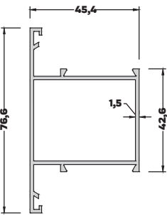
AL-245 (0,780 kg/mt) DAR ORTA KAYIT PROFİLİ
