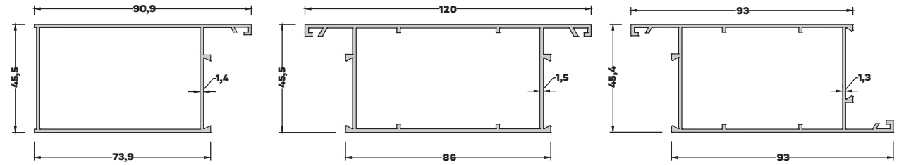
AL-2083 (0,986 kg/mt) BAZA KASA PROFİLİ
