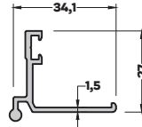
510-1103 (0,352 kg/mt) COTTA KÖŞE DÖNÜŞ PR. CMO3
