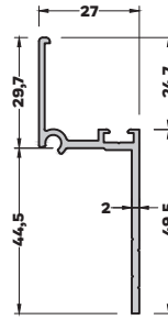
510-1104 (0,545 kg/mt) COTTA KÖŞE DÖNÜŞ PR. CMO4
