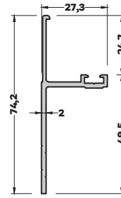
510-1105 (0,539 kg/mt) COTTA BİTİŞ PROFİLİ CMO5
