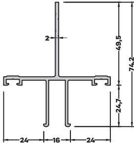
510-1101 (0,866 kg/mt) COTTA PROFİL CMO1
