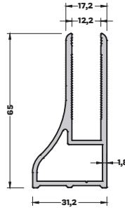
KHR40-1020 (1,063 kg/mt) 65'LİK YARIM CAM KANAL PROFİLİ
