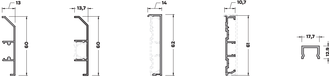
SP-4628 (0,317 kg/mt) SÜPÜRGELİK PROFİLİ
