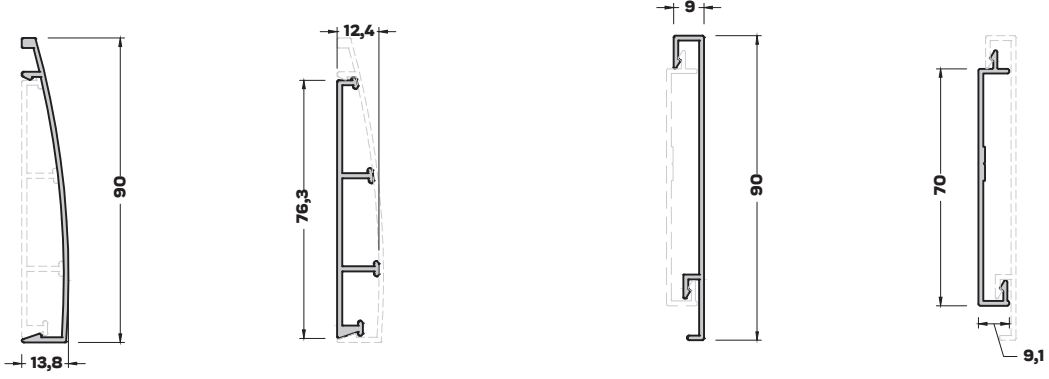
SP-4212 (0,433 kg/mt) SÜPÜRGELİK PROFİLİ
