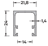
P-3621 (0,314 kg/mt) PANJUR YAN KASA PROFİLİ
