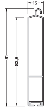
P-3046 (0,340 kg/mt) PANJUR ETEK PROFİLİ
