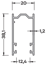
P-3195 (0,360 kg/mt) PANJUR YAN KASA PROFİLİ
