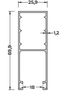
P-3991 (0,670 kg/mt) PANJUR YAN KASA PROFİLİ
