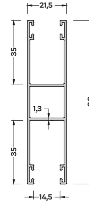
P-3420 (0,845 kg/mt) PANJUR ORTA KASA PROFİLİ
