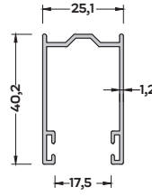
P-6163 (0,405 kg/mt) PANJUR YAN KASA PROFİLİ
