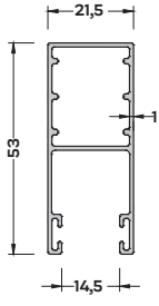
P-3872 (0,470 kg/mt) PANJUR YAN KASA PROFİLİ
