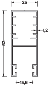
P-3730 (0,685 kg/mt) PANJUR YAN KASA PROFİLİ
