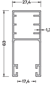
P-4061 (0,805 kg/mt) PANJUR YAN KASA PROFİLİ
