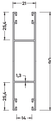
P-3419 (0,846 kg/mt) PANJUR ORTA KASA PROFİLİ
