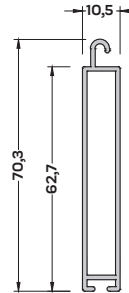
P-1901 (0,295 kg/mt) PANJUR ETEK PROFİLİ
