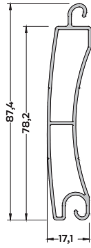
P-3946 (0,420 kg/mt) PANJUR LAMEL PROFİLİ
