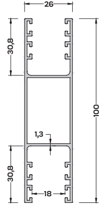
P-3453 (1,111 kg/mt) PANJUR ORTA KASA PROFİLİ
