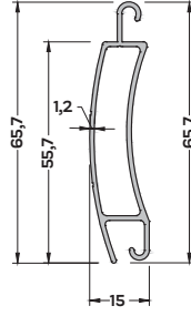
P-4871 (0,493 kg/mt) PANJUR LAMEL PROFİLİ
