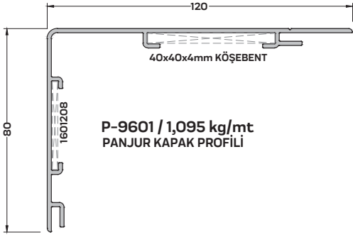
P-9601 (1,095 kg/mt) PANJUR KAPAK PROFİLİ
