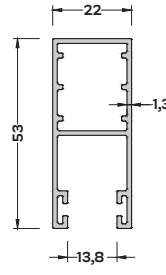
P-5042 (0,614 kg/mt) PANJUR YAN KASA PROFİLİ
