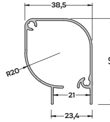
P-4073 (0,555 kg/mt) PANJUR PROFİLİ
