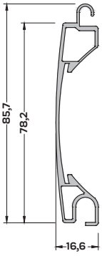
P-7056 (0,315 kg/mt) PANJUR LAMEL PROFİLİ
