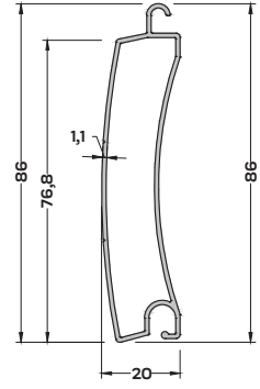
P-3430 (0,615 kg/mt) PANJUR LAMEL PROFİLİ
