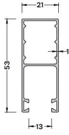
P-3948 (0,475 kg/mt) PANJUR YAN KASA PROFİLİ
