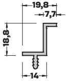
MB-5800 (0,238 kg/mt) ÇITA PROFİLİ
