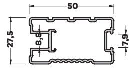
MB-5064 (0,446 kg/mt) ORTA BAĞLANTI PROFİLİ
