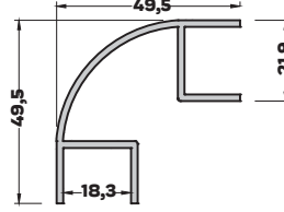
MB-5059 (0,745 kg/mt) BAZA DÖNÜŞ PROFİLİ
