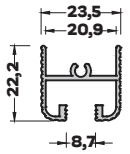
MB-5049 (0,295 kg/mt) ÜST BAĞLANTI PROFİLİ
