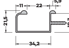
MB-5273 (0,410 kg/mt) KULP PROFİLİ
