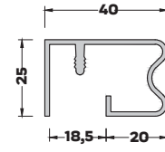
MB-3147 (0,530 kg/mt) BOY KULP PROFİLİ
