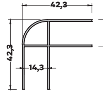
MB-5276 (0,472 kg/mt) BAZA DÖNÜŞ PROFİLİ
