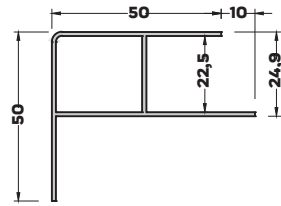
MB-5272 (0,582 kg/mt) BAZA KAPAMA PROFİLİ
