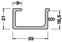
MB-5678 (0,590 kg/mt) KULP PROFİLİ
