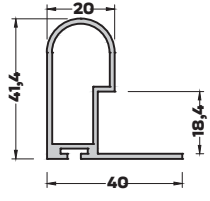
MB-5036 (0,583 kg/mt) BOY KULP PROFİLİ
