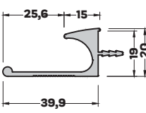
MB-5196 (0,534 kg/mt) KULP PROFİLİ
