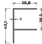
MB-6671 (0,263 kg/mt) BAZA KAPAMA PROFİLİ
