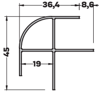
MB-4870 (0,488 kg/mt) BAZA DÖNÜŞ PROFİLİ
