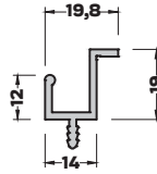
MB-5843 (0,295 kg/mt) ÇITA PROFİLİ
