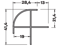
MB-5598 (0,410 kg/mt) BAZA DÖNÜŞ PROFİLİ
