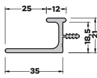
MB-5679 (0,485 kg/mt) KULP PROFİLİ
