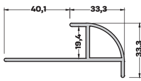
MB-4728 (0,788 kg/mt) BAZA KAPAMA PROFİLİ
