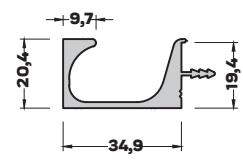
MB-5042 (0,652 kg/mt) KULP PROFİLİ
