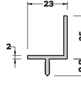
MB-5443 (0,306 kg/mt) ÇITA PROFİLİ
