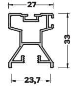
MB-7687 (0,498 kg/mt) YAN KULP PROFİLİ
