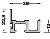
MB-8354 (0,436 kg/mt) YAN KULP PROFİLİ
