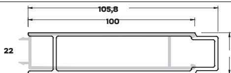
L-1249 (0,689 kg/mt) LAMBRI PROFİLİ
