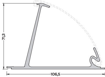
S-10068 (0,954 kg/mt) GÜNEŞ KIRICI PR.
