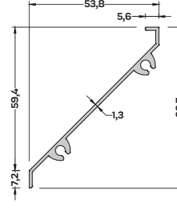
M-3164 (0,477 kg/mt) MENFEZ PROFİLİ
