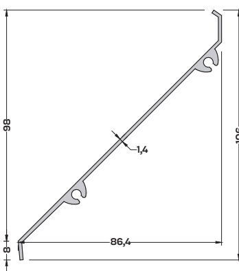
M-3757 (0,720 kg/mt) MENFEZ PROFİLİ
