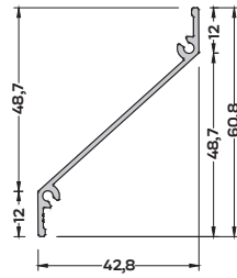
M-3076 (0,343 kg/mt) MENFEZ PROFİLİ
