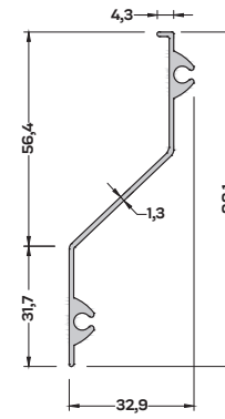
M-11031 (0,507 kg/mt) MENFEZ PROFİLİ
