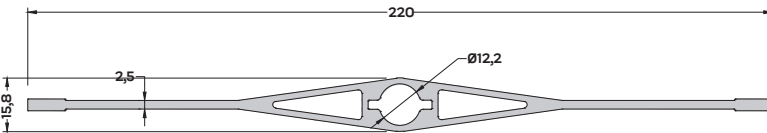
S-7348 (2,515 kg/mt) GÜNEŞ KIRICI PR. 200 mm
