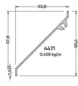
M-4471 (0,405 kg/mt) MENFEZ PROFİLİ
