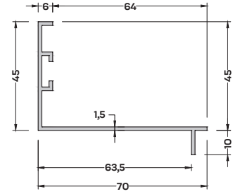
SC-906 KILAVUZ
