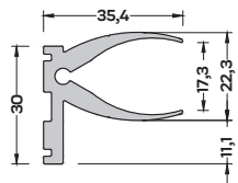
S-6745 (0,811 kg/mt) GÜNEŞ KIRICI AYAK PR.
