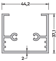
M-8905 (2,150 kg/mt) ÜST RAY PROFİLİ
