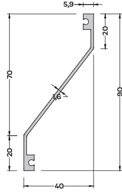
M-5382 (0,607 kg/mt) MENFEZ PROFİLİ
