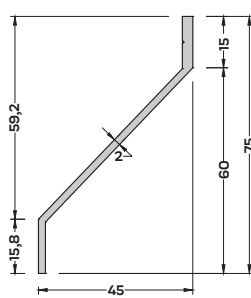
M-5297 (0,538 kg/mt) MENFEZ PROFİLİ
