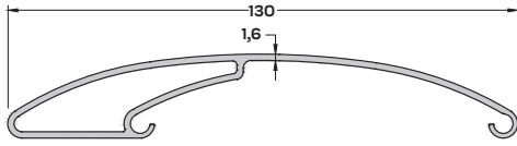
S-4000 (1,905 kg/mt) GÜNEŞ KIRICI PR.
