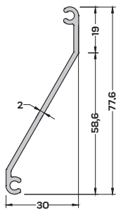
M-2815 (0,521 kg/mt) MENFEZ PROFİLİ
