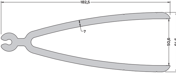
S-4005 (6,840 kg/mt) GÜNEŞ KIRICI TAŞIYICI AYAK PR.
