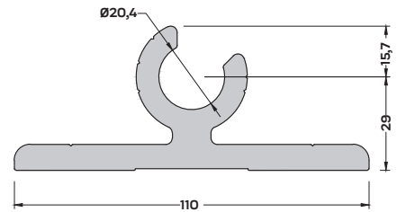
S-7523 (1,687 kg/mt) GÜNEŞ KIRICI AYAK PR.
