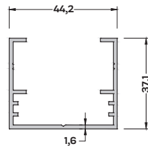
M-11096 (1,365 kg/mt) ÜST RAY PROFİLİ
