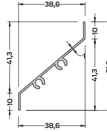
SC-905 KILAVUZ
