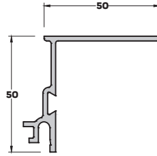
DL-2781 (0,708 kg/mt) DİLATASYON PROFİLİ
