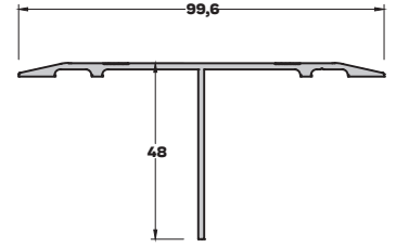
DL-8047 (0,707 kg/mt) DİLATASYON PROFİLİ
