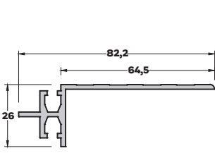
DL-3840 (0,700 kg/mt) DİLATASYON PROFİLİ
