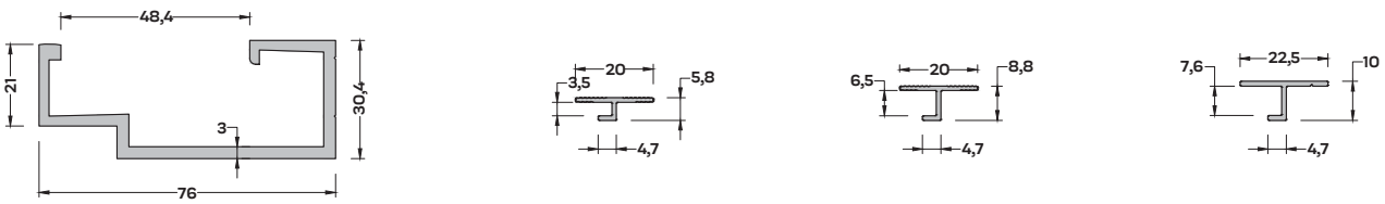
CK-6998 (1,208 kg/mt) KOMPAKT PROFİLİ
