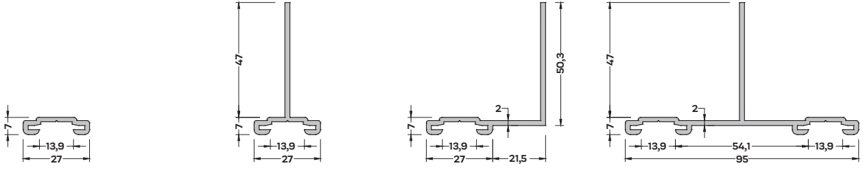
CK-4289 (0,226 kg/mt) SERAMİK CEPHE PR. 4289
