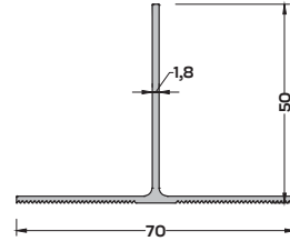
CK-6702 (0,528 kg/mt) T PROFİLİ
