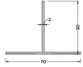
CK-6754 (0,601 kg/mt) T PROFİLİ
