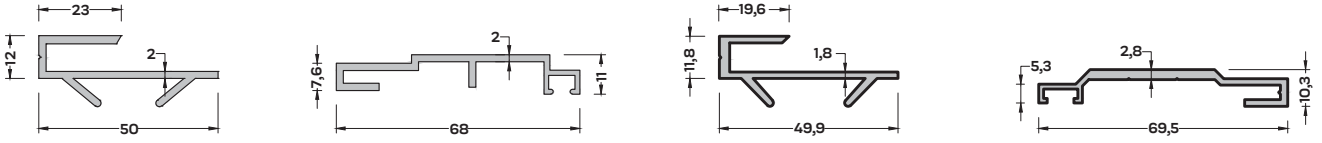
CK-4065 (0,577 kg/mt) SERMİK ALT BAĞLANTI PR.
