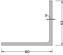
CK-4298 (0,899 kg/mt) L ANKRAJ PROFİLİ
