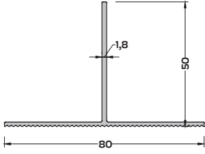
CK-6312 (0,531 kg/mt) T PROFİLİ
