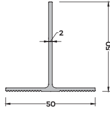
CK-6755 (0,507 kg/mt) T PROFİLİ
