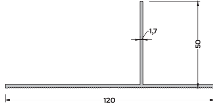
CK-6755 (0,507 kg/mt) T PROFİLİ
