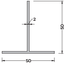
CK-6312 (0,531 kg/mt) T PROFİLİ
