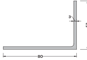
CK-4297 (1,062 kg/mt) L ANKRAJ PROFİLİ
