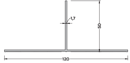
CK-6754 (0,601 kg/mt) T PROFİLİ
