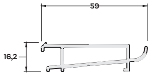
900-1201 (0,515 kg/mt) GOLD DUVAR BİTİM PROFİLİ
