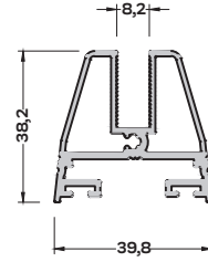
900-2104 (0,866 kg/mt) FIRTINA KANAT PR. 8 MM
