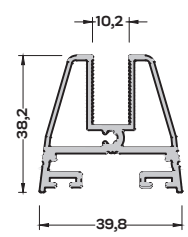
900-2105 (0,866 kg/mt) FIRTINA KANAT PR. 10 MM
