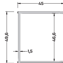
900-6105 (0,554 kg/mt) GOLD SERİ AYAR PROFİLİ
