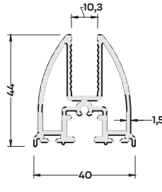
900-2102 (0,991 kg/mt) GOLD KANAT PR. 10 MM
