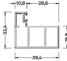
900-1202 (0,544 kg/mt) FIRTINA DUVAR BİTİM PROFİLİ
