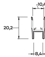
900-6101 (0,169 kg/mt) 8 MM H PROFİLİ
