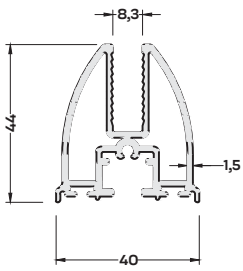
900-2101 (0,993 kg/mt) GOLD KANAT PR. 8 MM
