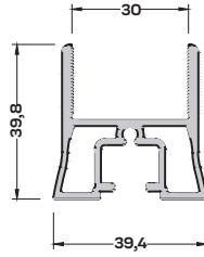
900-2103 (0,874 kg/mt) GOLD KANAT PR.30 MM
