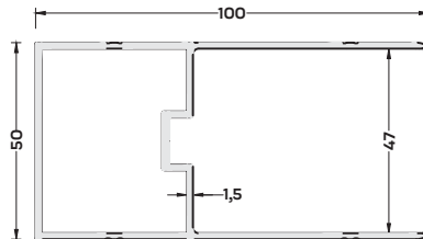
900-6104 (1,248 kg/mt) GOLD SERİ AYAR PROFİLİ
