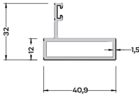
900-1201 (0,515 kg/mt) GOLD DUVAR BİTİM PROFİLİ
