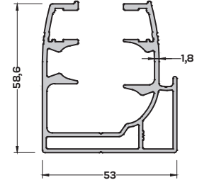
900-1102 (1,548 kg/mt) FIRTINA KASA PROFİLİ
