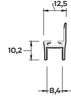
900-6102 (0,142 kg/mt) 8 MM U PROFİLİ
