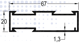
TB-3020 / 0,715 kg/mt SÜRME KASA PROFİLİ
