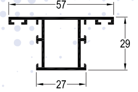
TB-3028 / 0,631 kg/mt ORTA KAYIT PROFİLİ
