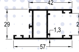
TB-3021 / 0,680 kg/mt SÜRME KANAT PROFİLİ
