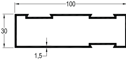
TB-3030 / 1,151 kg/mt SÜRME KASA PROFİLİ
