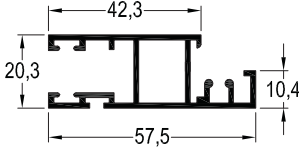
TB-3711 / 0,711 kg/mt SİNEKLİK KANAT PROFİLİ
