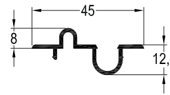
TB-3029 / 0,289 kg/mt 4'LÜ KANAT "S" KAPAK PROFİLİ
