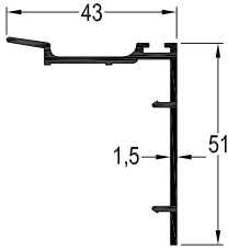
TB-3033 / 0,444 kg/mt KENET KAPAK PROFİLİ
