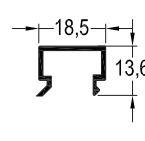
TB-3179 / 0,156 kg/mt ÜST RAY PROFİLİ
