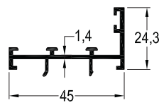
TB-3032 / 0,413 kg/mt ADAPTÖR PROFİLİ
