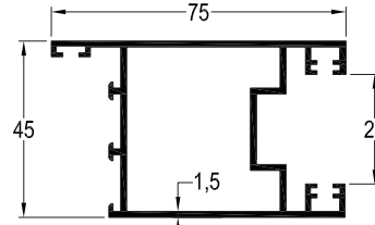
TB-3031 / 1,161 kg/mt SÜRME KANAT PROFİLİ
