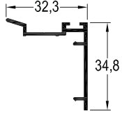
TB-3023 / 0,267 kg/mt KENET KAPAK PROFİLİ
