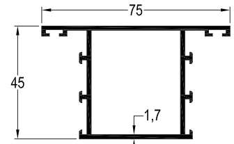
TB-2252 / 1,062 kg/mt GENİŞ ORTA KAYIT PROFİLİ
