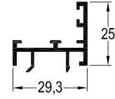
TB-3022 / 0,333 kg/mt ADAPTÖR PROFİLİ
