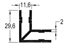
TB-1221 / 0,594 kg/mt KÖŞE ÇAVUŞ BAĞLANTI
