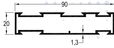
TB-3710 / 0,946 kg/mt SİNEKLİKLİ SÜRME KASA PROFİLİ
