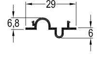
TB-3027 / 0,150 kg/mt 4'LÜ KANAT "S" KAPAK PROFİLİ
