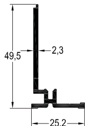
SP-6433 / 0,452 kg/mt SÜPÜRGELİK ALT PROFİLİ
