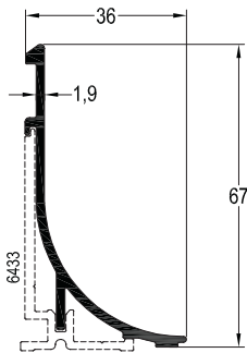
SP-6432 / 0,542 kg/mt SÜPÜRGELİK PROFİLİ
