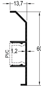
SP-4207 / 0,328 kg/mt SÜPÜRGELİK PROFİLİ
