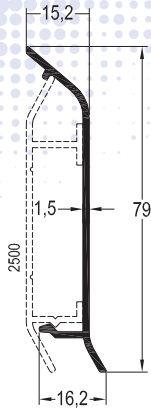
SP-2501 / 0,400 kg/mt SÜPÜRGELİK PROFİLİ
