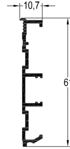
SP-5327 / 0,377 kg/mt SÜPÜRGELİK ALT PROFİLİ
