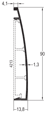
SP-4512 / 0,433 kg/mt SÜPÜRGELİK PROFİLİ
