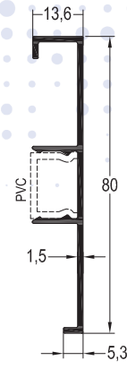
SP-5477 / 0,501 kg/mt SÜPÜRGELİK PROFİLİ
