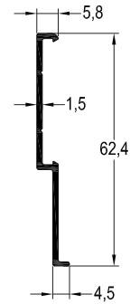
SP-5690 / 0,295 kg/mt SÜPÜRGELİK ALT PROFİLİ
