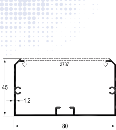
SP-3736 / 0,744 kg/mt KABLO KANALLI SÜPÜRGELİK
