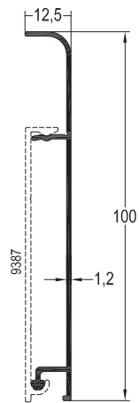
SP-9387 / 0,444 kg/mt SÜPÜRGELİK PROFİLİ
