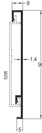
SP-5296 / 0,460 kg/mt SÜPÜRGELİK PROFİLİ
