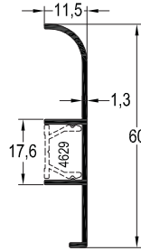
SP-4628 / 0,154 kg/mt SÜPÜRGELİK PROFİLİ
