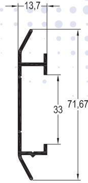
SP-2500 / 0,450 kg/mt SÜPÜRGELİK ALT PROFİLİ
