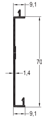
SP-5477 / 0,501 kg/mt SÜPÜRGELİK PROFİLİ
