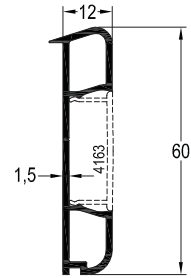
SP-4510 / 0,488 kg/mt SÜPÜRGELİK PROFİLİ
