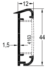
SP-4164 / 0,332 kg/mt SÜPÜRGELİK PROFİLİ
