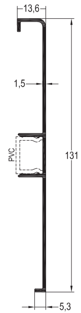
SP-6271 / 0,703 kg/mt SÜPÜRGELİK PROFİLİ
