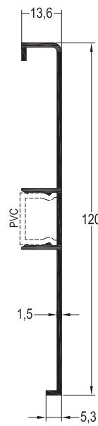
SP-4295 / 0,660 kg/mt SÜPÜRGELİK PROFİLİ
