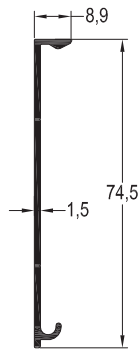
SP-9386 / 0,357 kg/mt SÜPÜRGELİK ALT PROFİLİ
