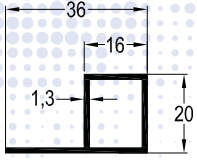
SN-3277 / 0,309 kg/mt İÇE AÇILIR SİNEKLİK KASA PROFİLİ
