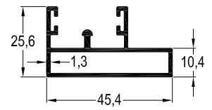
SN-5374 / 0,588 kg/mt SİNEKLİK PROFİLİ
