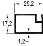
SN-4107 / 0,282 kg/mt SİNEKLİK PROFİLİ
