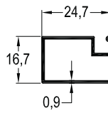
SN-5967 / 0,222 kg/mt SİNEKLİK PROFİLİ
