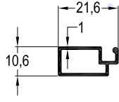
SN-2119 / 0,170 kg/mt SİNEKLİK PROFİLİ
