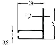
SN-1437 / 0,316 kg/mt SİNEKLİK F PROFİLİ
