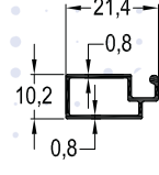
SN-6056 / 0,138 kg/mt SİNEKLİK PROFİLİ
