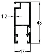
SN-10809 / 0,460 kg/mt SÜRME SİNEKLİK PROFİLİ
