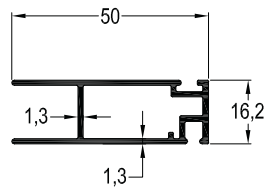
SN-5372 / 0,503 kg/mt SİNEKLİK SÜRME KANAT PROFİLİ
