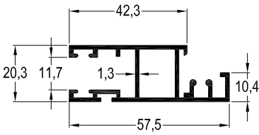
SN-3711 / 0,774 kg/mt SİNEKLİK SÜRME KANAT PROFİLİ
