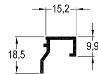
SN-3712 / 0,172 kg/mt SİNEKLİK ÇİTA PROFİLİ
