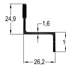
SN-10807 / 0,330 kg/mt SİNEKLİK RAY PROFİLİ
