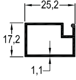
SN-1444 / 0,261 kg/mt SİNEKLİK PROFİLİ
