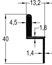
SN-2285 / 0,370 kg/mt SİNEKLİK RAY PROFİLİ
