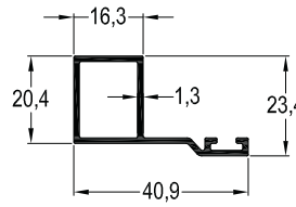
SN-5478 / 0,361 kg/mt SİNEKLİK PROFİLİ
