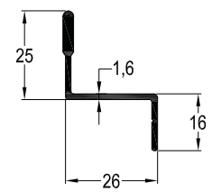
SN-5373 / 0,316 kg/mt SİNEKLİK RAY PROFİLİ
