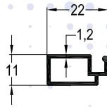
SN-4106 / 0,207 kg/mt SİNEKLİK PROFİLİ
