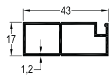
SN-4108 / 0,442 kg/mt SİNEKLİK PROFİLİ
