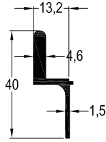
SN-454 / 0,384 kg/mt SİNEKLİK RAY PROFİLİ
