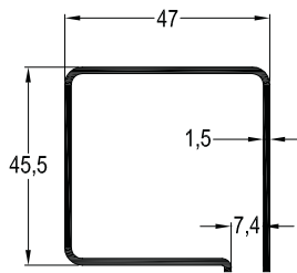
SN-1436 / 0,688 kg/mt SİNEKLİK PROFİLİ
