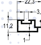
SN-1459 / 0,206 kg/mt SİNEKLİK PROFİLİ
