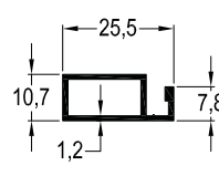
SN-1490 / 0,227 kg/mt SİNEKLİK PROFİLİ
