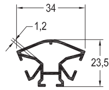
ST-317 / 0,430 kg/mt
