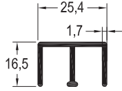
ST-177 / 0,327 kg/mt SÜRME E PROFİLİ
