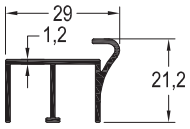
ST-4657 / 0,287 kg/mt SÜRME KUYRUKLU E PROFİLİ
