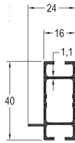
ST-2556 / 0,427 kg/mt
