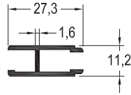
ST-5091 / 0,269 kg/mt SEHPA H PROFİLİ
