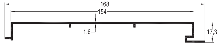
L-4426 / 0,925 kg/mt LAMBRI PROFİLİ
