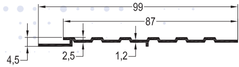
L-222 / 0,378 kg/mt LAMBRI PROFİLİ
