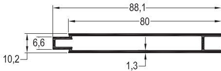
L-1249 / 0,689 kg/mt LAMBRI PROFİLİ
