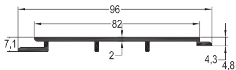
L-2000/20 / 0,635 kg/mt LAMBRI PROFİLİ
