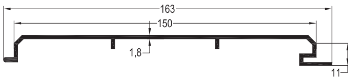
L-1640 / 0,998 kg/mt LAMBRI PROFİLİ
