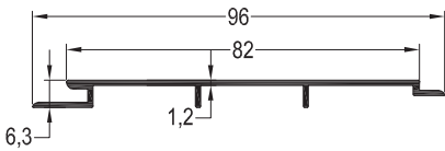
L-2000/12 / 0,395 kg/mt LAMBRI PROFİLİ
