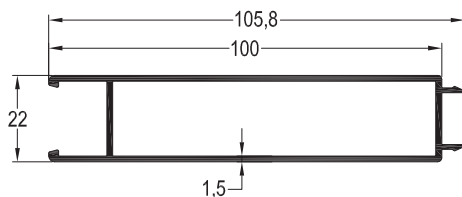
L-785 / 1,017 kg/mt LAMBRI PROFİLİ
