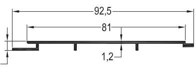
L-1317 / 0,362 kg/mt LAMBRI PROFİLİ
