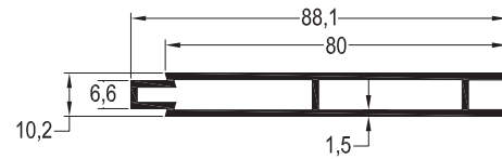
L-2639 / 0,810 kg/mt LAMBRI PROFİLİ
