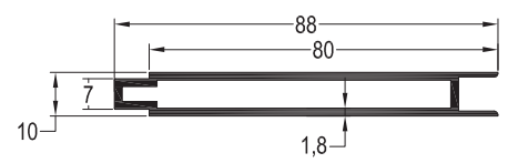
L-4442 / 0,886 kg/mt LAMBRI PROFİLİ
