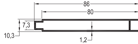
L-115 / 0,609 kg/mt LAMBRI PROFİLİ
