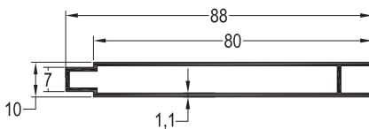
L-3010 / 0,570 kg/mt LAMBRI PROFİLİ
