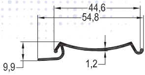
L-124 / 0,237 kg/mt LAMBRI PROFİLİ
