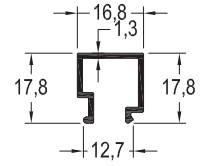
FS-4136 / 0,203 kg/mt CAM ÇİTA PROFİLİ
