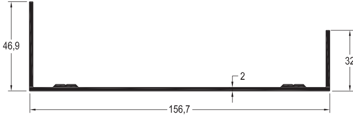
FS-4120 / 1,360 kg/mt MEKANİZMA KAPAK PROFİLİ
