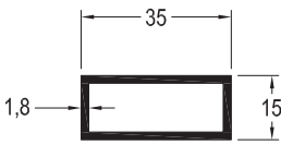
FS-4142 / 0,453 kg/mt KUTU PROFİLİ
