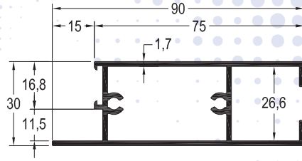
FS-4139 / 1,198 kg/mt ÜST ETEK PROFİLİ
