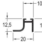
FS-4137 / 0,153 kg/mt ÜST KAPAK PROFİLİ
