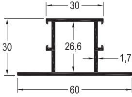
FS-4138 / 0,585 kg/mt KANAT PROFİLİ
