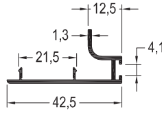
FS-4135 / 0,276 kg/mt YAN KAPAK PROFİLİ
