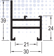
FS-4138 / 0,585 kg/mt KANAT PROFİLİ
