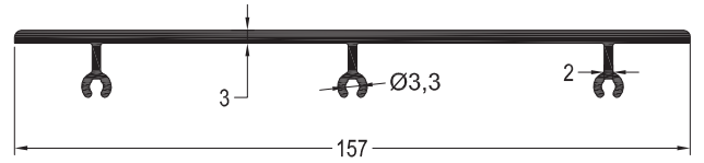
FS-4121 / 1,562 kg/mt BAĞLANTI PROFİLİ
