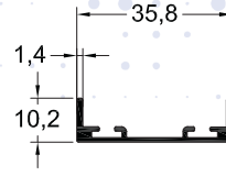
AS-1818 / 0,224 kg/mt DUVAR BİTİM PROFİLİ
