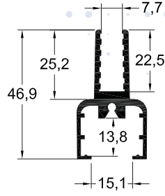
AS-1816 / 0,699 kg/mt KANAT PROFİLİ
