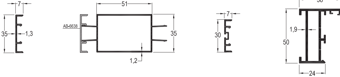
AB-6638 (0,203 kg/mt) KAPAK PROFİLİ
