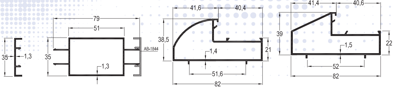
AB-1844 (0,197 kg/mt) KAPAK PROFİLİ
