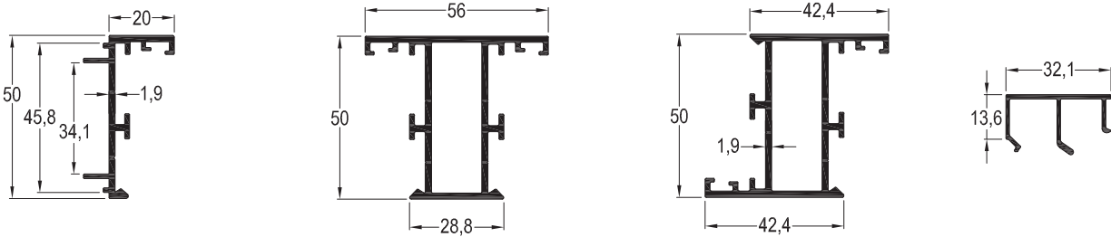
AB-6541 (0,556 kg/mt) ADAPTÖR PROFİLİ
