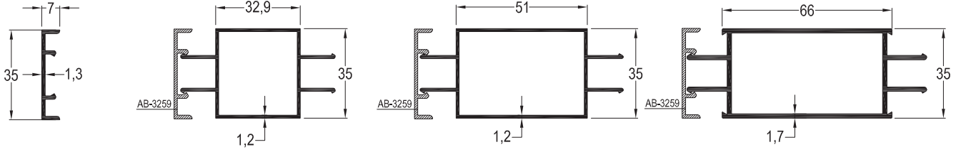
AB-3259 (0,200 kg/mt) KAPAK PROFİLİ
